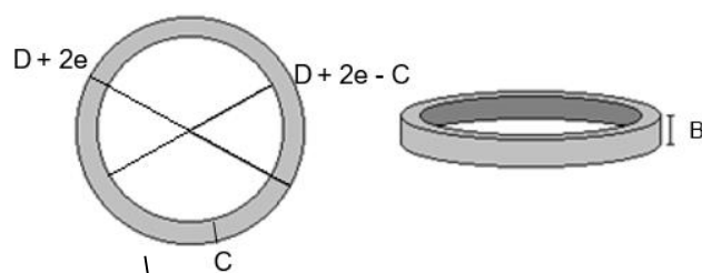
Figura 5 - Esquema de uma coroa cilíndrica
