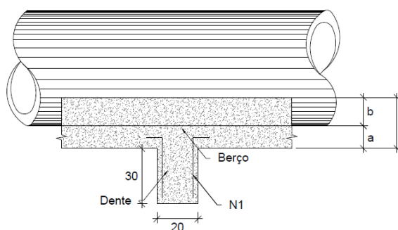
Figura 6 - Representação do dente de concreto
