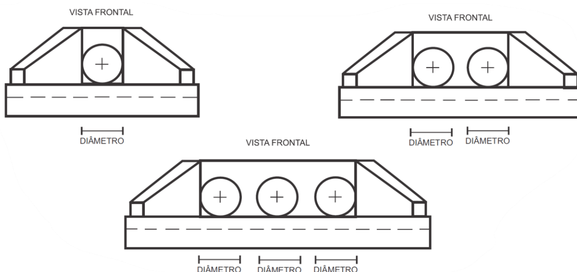
Figura 3 - Bocas de bueiros tubulares simples, duplos e triplos
